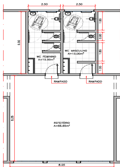
PLANTA BAIXA – SITUAÇÃO ATUAL ESC.: 1:100
