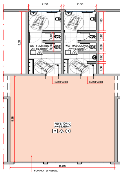
PLANTA BAIXA – SITUAÇÃO PRETENDIDA ESC.: 1:100
