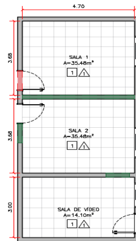
PLANTA BAIXA – SITUAÇÃO PRETENDIDA ESC.: 1:100
